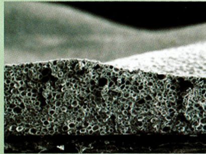
塗膜断面拡大写真
